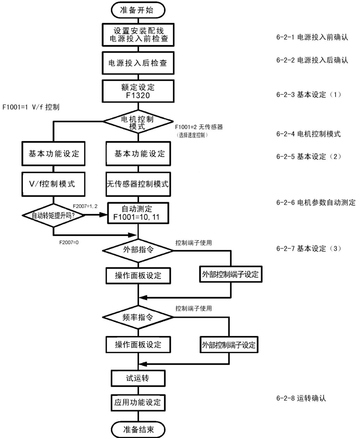
图 6-1 运转步骤流程
