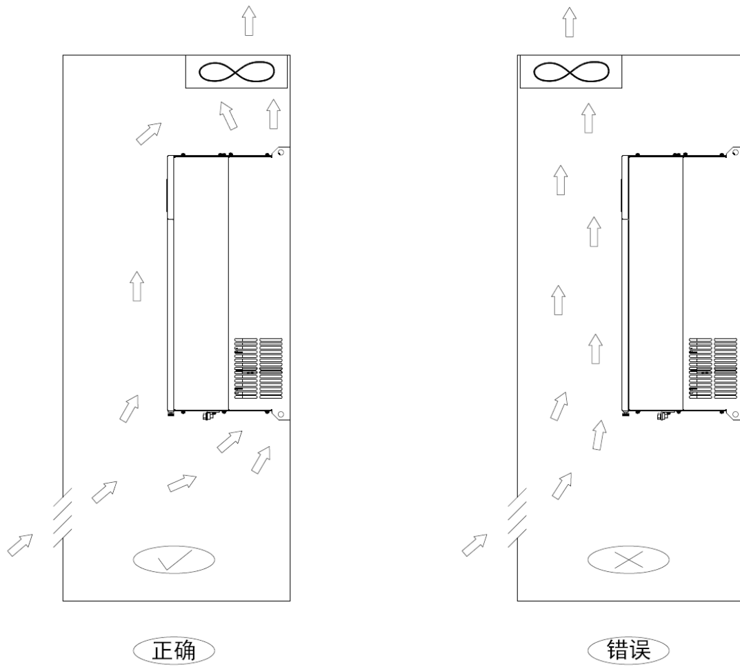
图 3-2 柜内换气扇的安装位置
