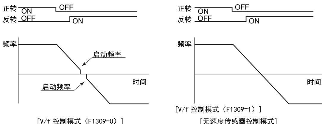
图 6-2 外部运转指令动作
