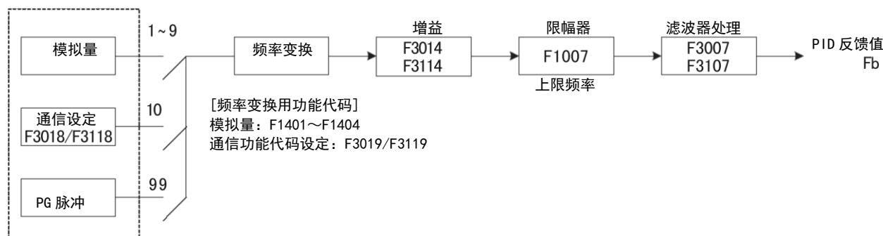
PID 反馈输入切换 F3002/F3102
