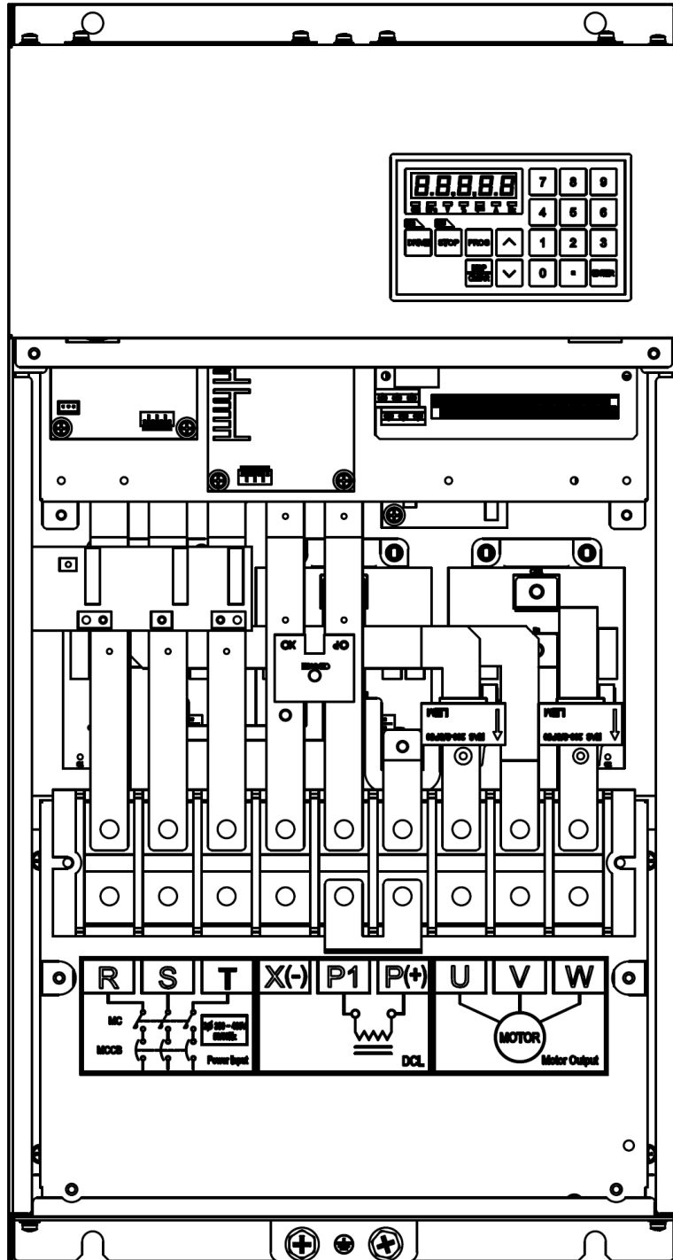
拆卸下面盖完成后的示意图
