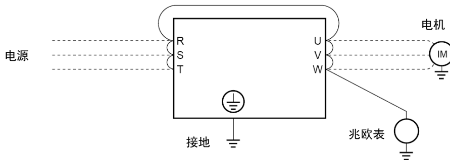
图 10-6 兆欧表测试电路图
